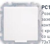
ТРК-004 Розетка комбинированная (телефонная + компьютерная) 73x73x36,8
